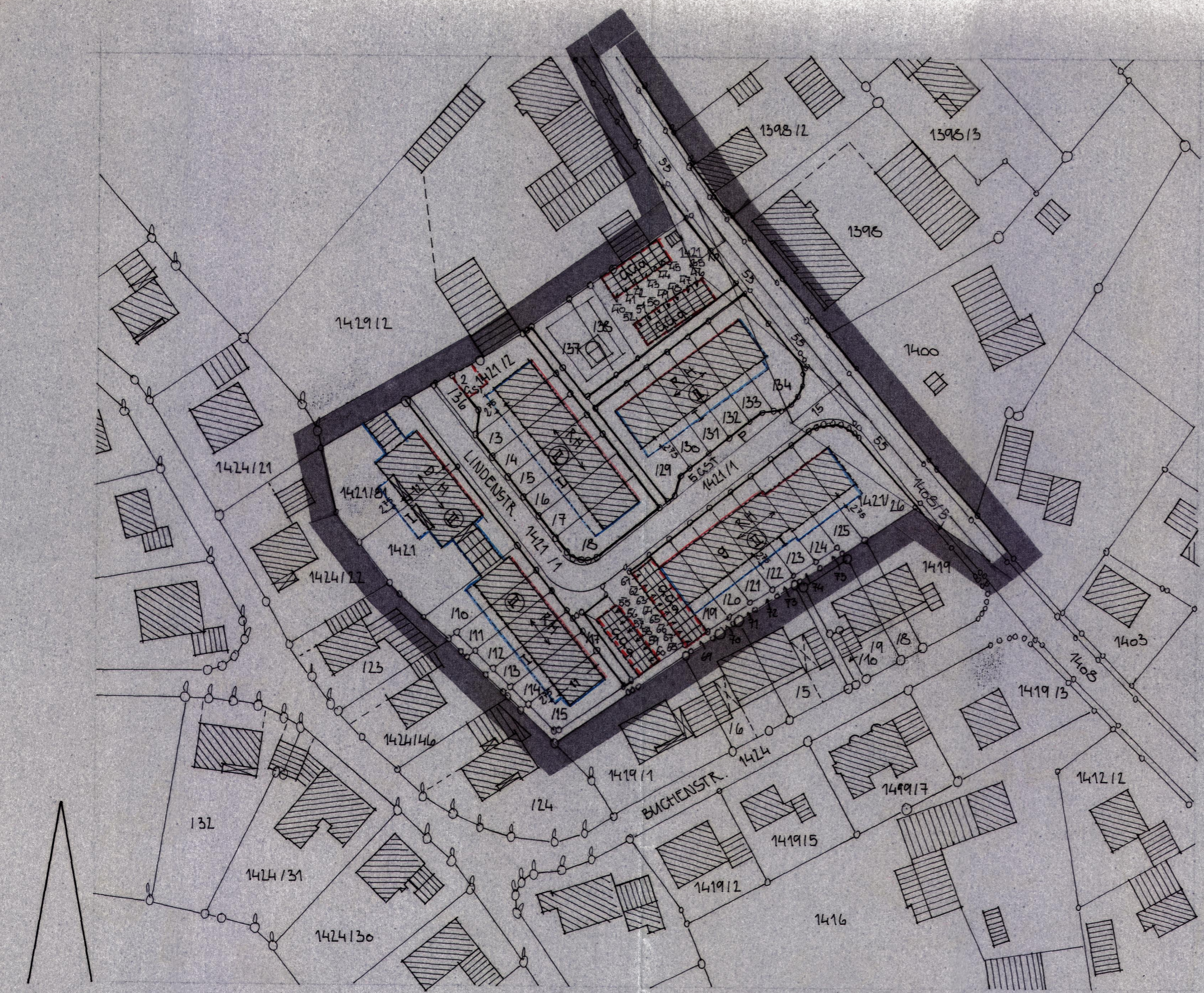
LAGEPLAN M · 1 : 1000
